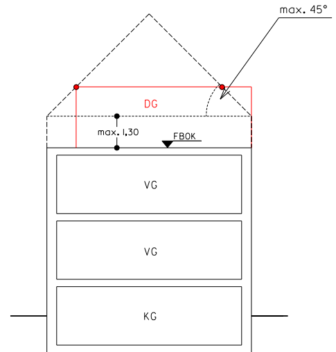
Schnitt 1
